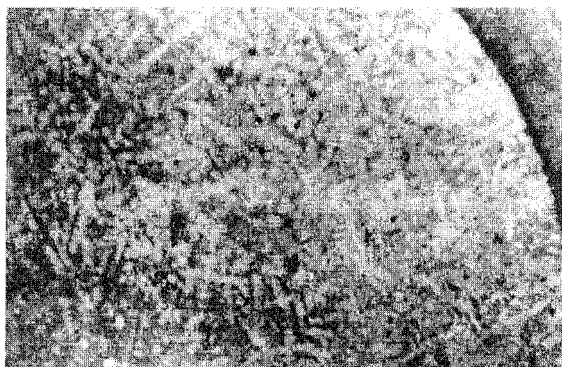
Slika 6 - Poprečni presek kristala. Sitnozrni deo klice na rastojanju 10 mm od početka. (uveličanje 24x)
