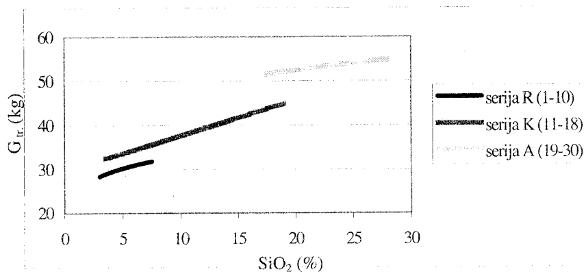
Slika 5 - Količina dobijene troske u funkciji sadržaja MnO_2 (%) Figure 5 - Slag quantity as a function of MnO_2 content (%)
