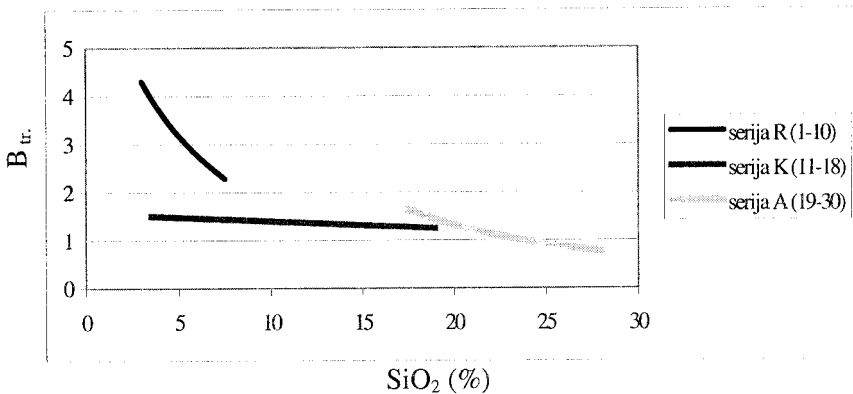
Slika 8 - Bazicitet troske u zavisnost od sadržaja SiO_2 (%) Figure 8 - Basicity of slag as a function of SiO_2 content (%)
